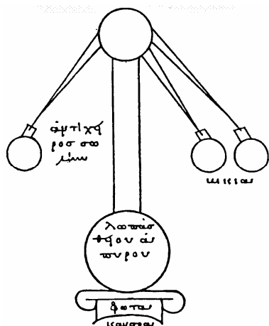
τρίβικος αποστακτήρας
